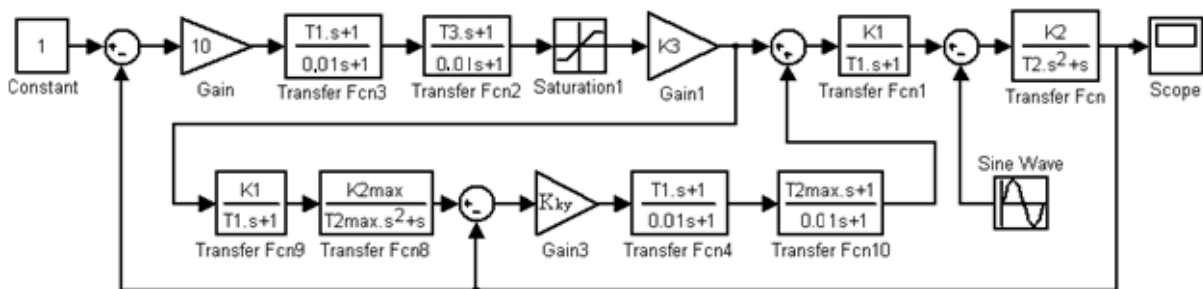
Рис.5. Схема модели системы в пакете Simulink
