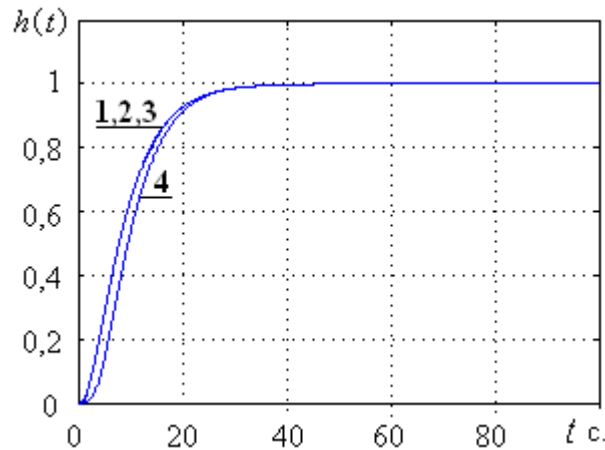
Рис. 6. Переходные характеристики при различных значениях параметров объекта: 1 – K_2 = 0,12; T_2 = 140\text{с.} ; 2 – K_2 = 0,12; T_2 = 14\text{с.} ; 3 – K_2 = 0,012; T_2 = 14\text{с.} ; 4 – K_2 = 0,012; T_2 = 140\text{с.}
